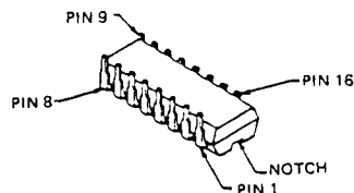
MC14518BCP (Q2002)
