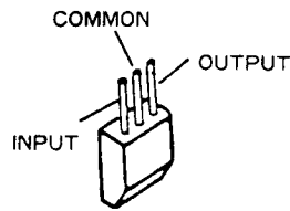
μPC78L05 (Q7010)
