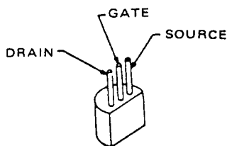
2SK125 (Q1005,1007)
