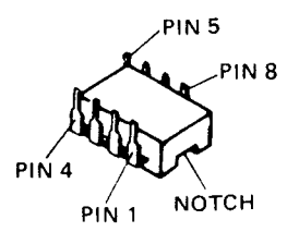
μPB571C (Q2008)
