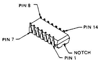
MC14066BCP (Q1038, 1055)
